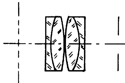
Ortoscopico di Plössl (Or) \sim 50^\circ
