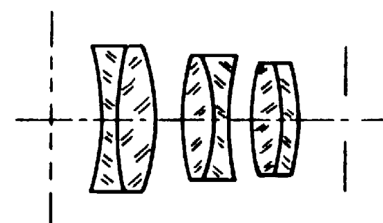
Erfle a 6 lenti (Er) \sim 70^\circ
