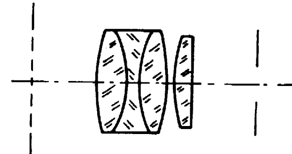
Ortoscopico di Abbe (Or) \sim 40^\circ
