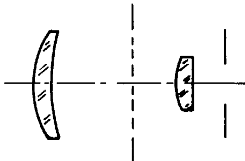
Huygens Mittenzwey (HM) \sim 45^\circ
