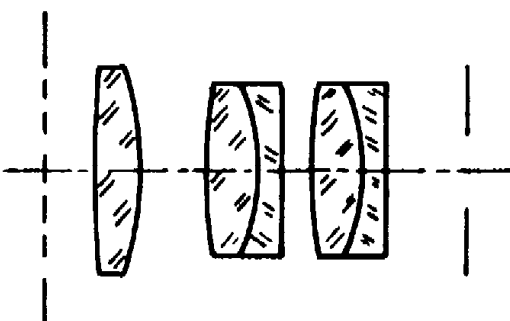
Erfle a 5 lenti (Er) \sim 65^\circ
