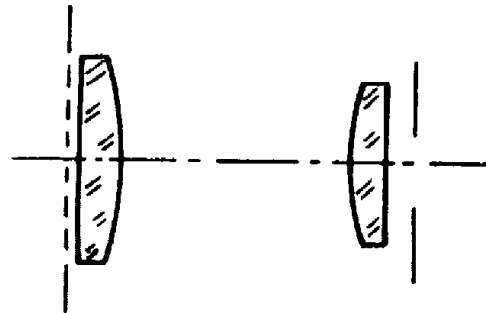
Huygens (H) \sim 35^\circ
