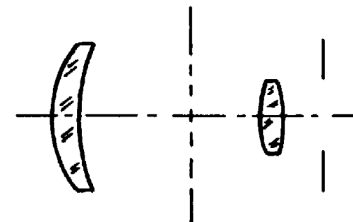
Huygens-Airy \sim 45^\circ
